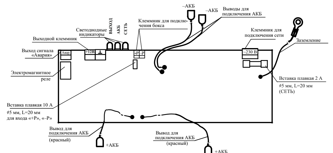
Рисунок 1 – Плата источника
